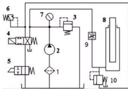
1. 滤油器 2. 叶片泵 3. 溢流阀 4. 电磁换向阀 5. 行程滑阀 6. 压力继电器 7. 压力表 8. 柱塞缸 9. 节流阀 10. 液控顺序阀
