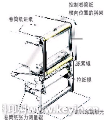
图1 纸带张力预置装置
