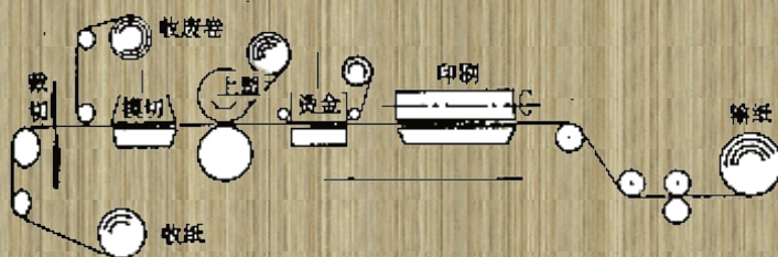
图6-6 不干胶标签印刷机结构示意图
