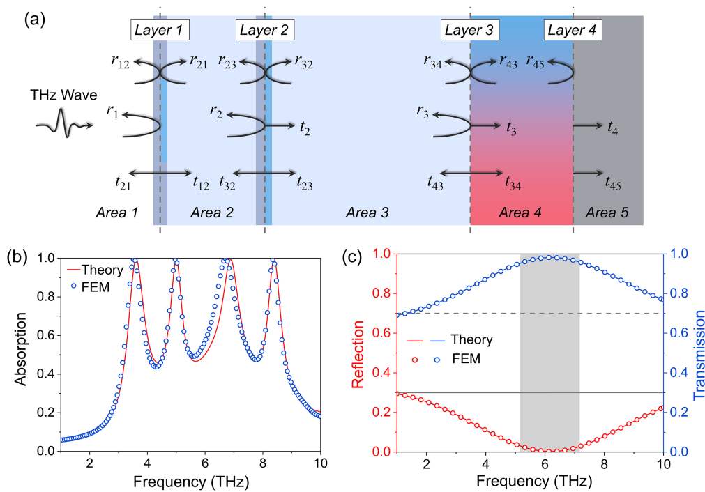
图2 (a) 所提出超构表面的多重反射干涉理论模型示意图；(b) 当二氧化钛为金属态时，理论和仿真得到的吸收谱；(c) 当二氧化钛为介质态时，理论和仿真得到的透射谱和反射谱。
