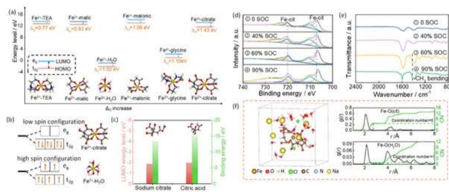
图1 (a-c) 配体量子化学计算筛选；(d-e) XPS与FTIR分析；(f) \text{Fe}^{2+} -citrate络合物溶剂化结构DFT-MD计算
