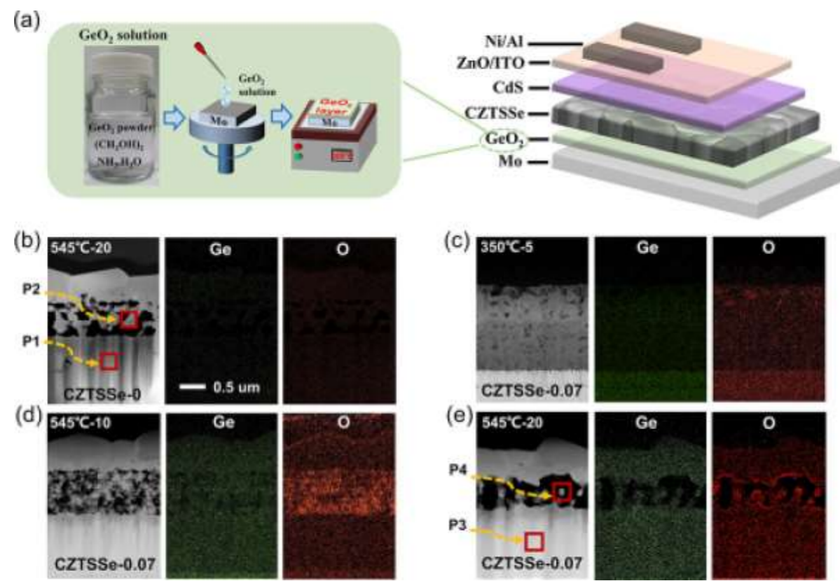
图1 (a) 旋涂法制备GeO 2 层及CZTSSe器件结构示意图； CZTSSe-0-GeO 2 和CZTSSe-0.07-GeO 2 薄膜中Ge和O元素在不同硒化条件下的STEM-EDS扫描图： (b) CZTSSe-0-GeO 2 薄膜在545°C-20, (c) CZTSSe-0.07-GeO 2 薄膜在350°C-5, (d) CZTSSe-0.07-GeO 2 薄膜在545°C-10, (e) CZTSSe-0.07-GeO 2 薄膜在545°C-20。
