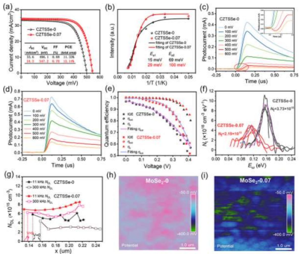
图2 (a) 基于CZTSSe-0-GeO 2 和CZTSSe-0.07-GeO 2 电池J-V曲线; CZTSSe-0-GeO 2 和CZTSSe-0.07-GeO 2 器件的缺陷及复合性质; (b)由稳态荧光谱得到的激活能E a ; (c)CZTSSe--0-GeO 2 样品的变偏压TPC; (d) CZTSSe--0.07-GeO 2 样品的变偏压TPC; (e) 基于TPC和TPV测试获得的收集效率η c 和抽取效率η ext ; (f) 基于导纳谱获得的缺陷态密度; (g) 基于DLCP表征获得载流子密度; (h) MoSe 2 -0-GeO 2 样品表面电势; (i) MoSe 2 -0.07-GeO 2 样品表面电势。
