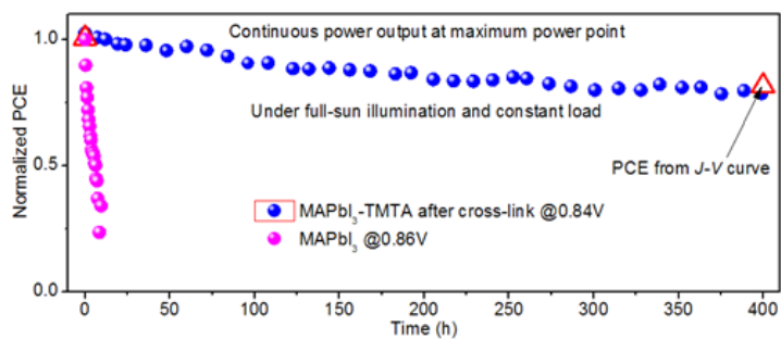
图2 基于原位交联策略的钙钛矿电池的连续功率输出（标准Xe灯光源，全光谱，恒定0.84V负载）
