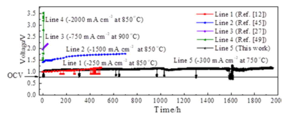
图1 CO 2 电解运行的长期稳定性
