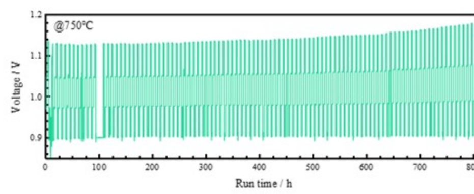
图3 脉冲循环CO 2 电解运行曲线
