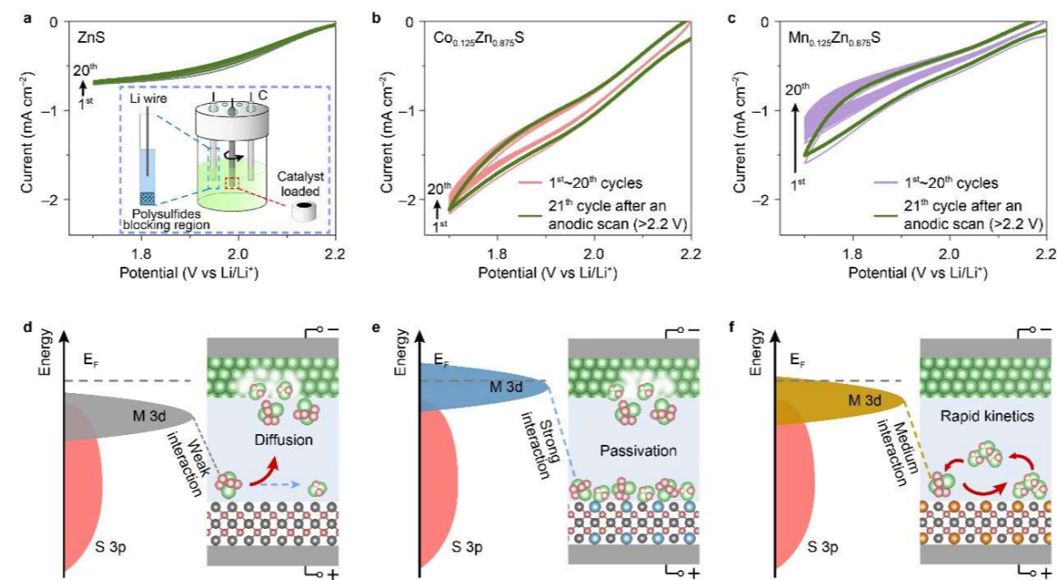
图3. 旋转圆盘电极表征催化剂钝化
