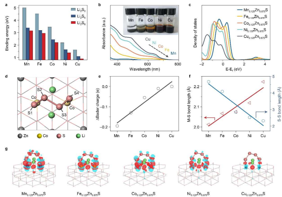
图2. 催化过程的机理研究
