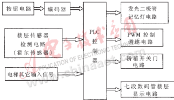
图2 电梯控制系统硬件结构框图
