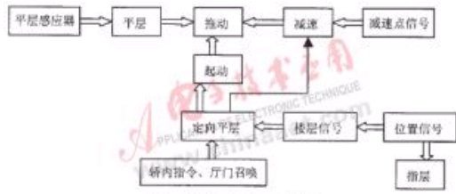
图1 电梯控制系统原理框图
