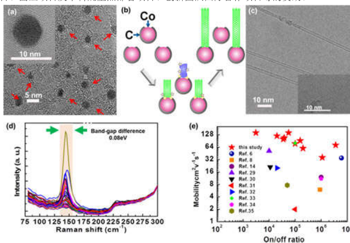
图 (a) 部分碳包覆Co催化剂的TEM照片; (b) 窄带隙分布半导体性SWCNT的生长示意图; (c) 所得SWCNT的TEM照片; (d) 所得半导体性SWCNT的激光拉曼光谱图(激光波长为532 nm); (e) 以所得SWCNT为沟道材料制备的薄膜晶体管的器件性能。
