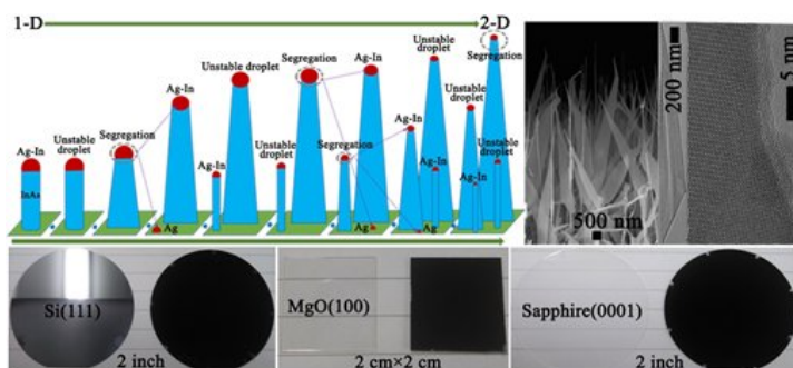
利用催化剂偏析技术实现了晶圆级高质量InAs纳米结构的维度调控
