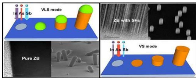
图2. InAsSb纳米线两种不同生长机制
