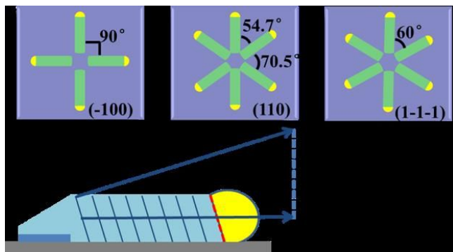
图3. 平面InAsSb纳米线在不同取向的Si衬底上方向分布及生长模型示意图
