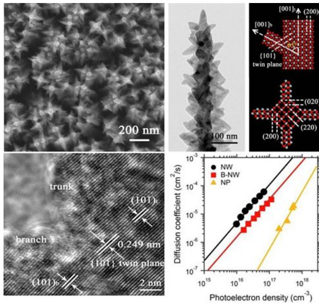
图1 具有快速电子传输性能的阵列二维枝状二氧化钛纳米电极。(Feng, X. J * Nano Lett. 2014, 14, 1848-1852.)
