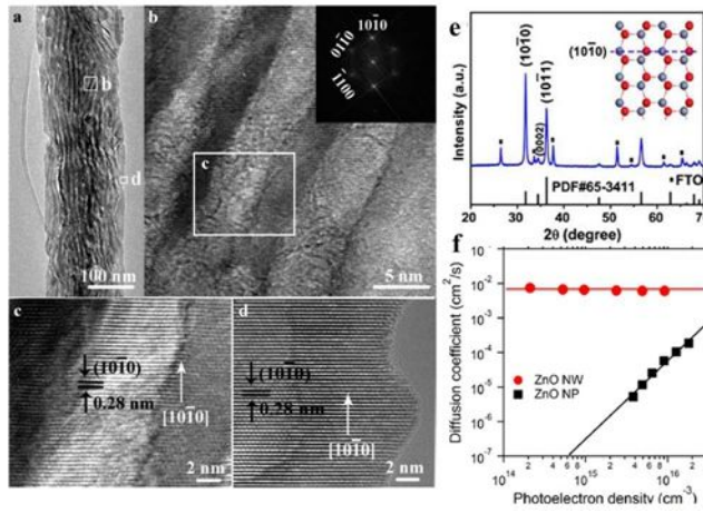
图2 具有快速电子传输性能及[10-10]生长方向的阵列多孔道氧化锌纳米电极。(Feng, X. J * J. Am. Chem. Soc. 2014, 136, 16772-16775.)
