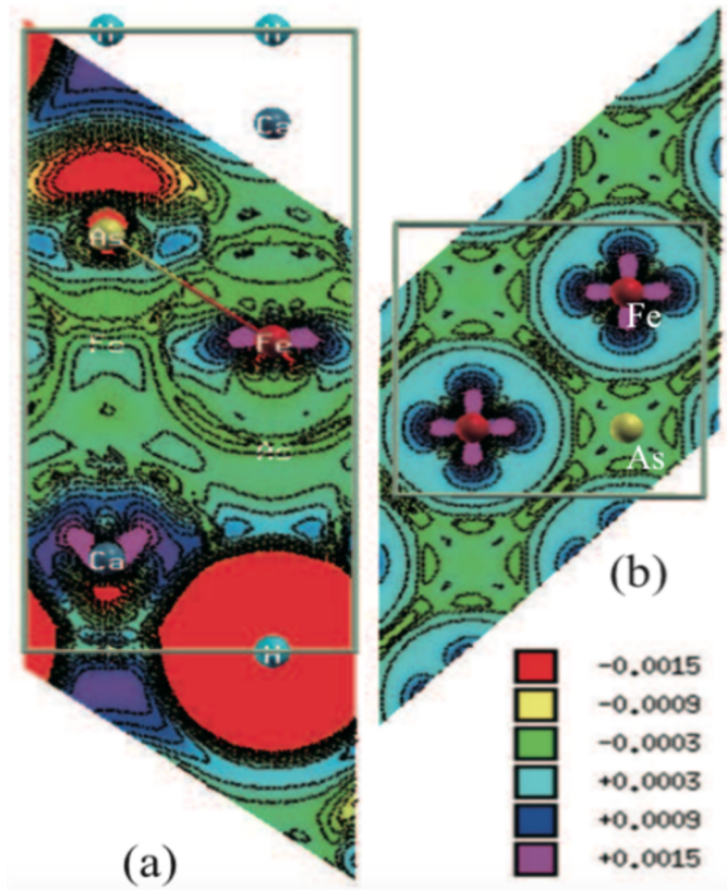
图2. 相同晶格参数下电荷密度差值 \rho(\text{CaFeAsH})-\rho(\text{CaFeAsF})
