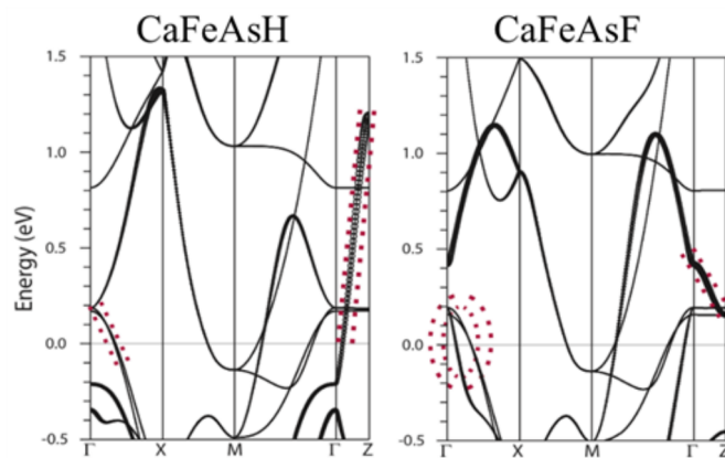
图1. As-4p z 轨道的特征能带图
