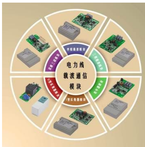
图2: 开发的多款电力线载波通信模块
