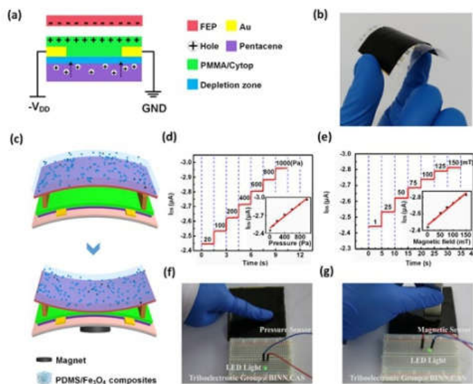
(a) 无栅极摩擦电子学晶体管工作原理示意图。(b) 用于力磁感应的无栅极柔性摩擦电子学晶体管实物图。(c) 力磁传感工作原理示意图。(d) 不同压力下源漏电流的变化。(e) 不同磁场强度下源漏电流的变化。(f) 手指按压传感器控制LED灯亮度演示压力传感。(g) 磁铁接近传感器控制LED灯亮度演示磁场强度传感。
