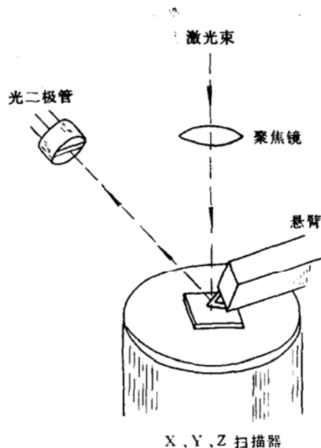
图 1b 用激光束测量弹性悬臂起伏的 AFM
