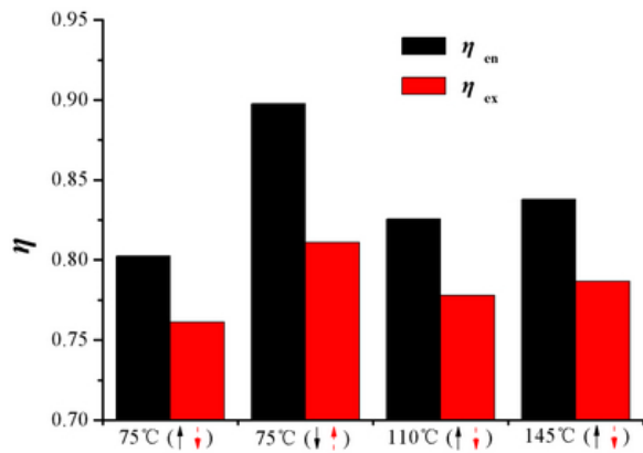
图3 不同工况下的储热效率和 效率
