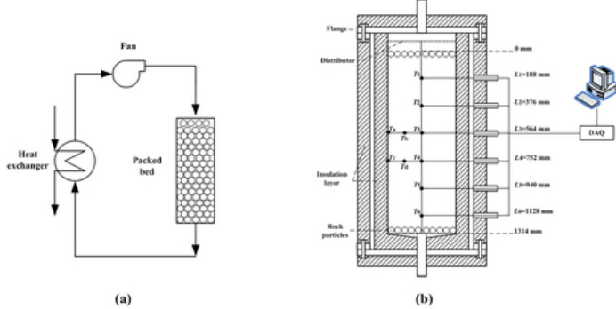
图1 新型间接式常压储热系统：(a)间接储热回路 (b)填充床储热装置
