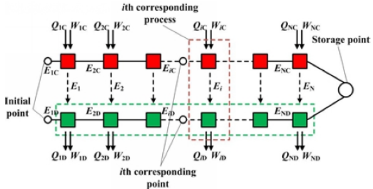
图1 对应点分析模型
