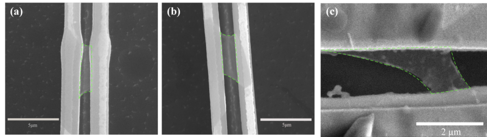
图1 用PMMA转移至电极的硫化钼薄膜
