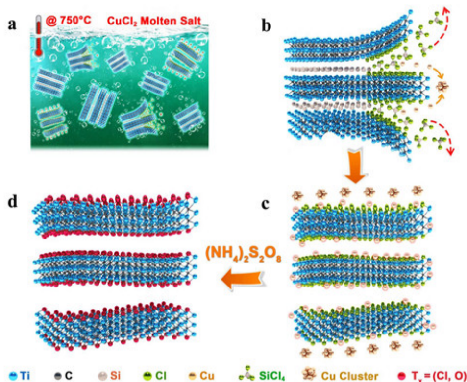
图1 路易斯酸熔盐合成MXene示意图：以CuCl 2 刻蚀Ti 3 SiC 2 合成Ti 3 C 2 T x MXene的示意图为例
