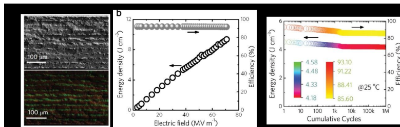
左: NBT-SBT多层陶瓷电容器截面SEM照片中、右: NBT-SBT多层陶瓷电容器储能特性实验测试结果、疲劳实验结果
