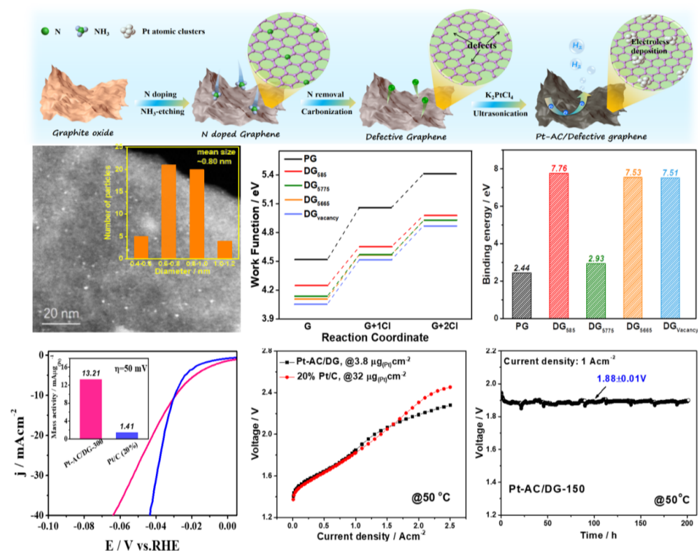
图1. 超小Pt-AC/DG制备流程、物理表征、DFT计算、电化学HER活性以及质子交换膜水电解器件稳态极化曲线和稳定性测试
