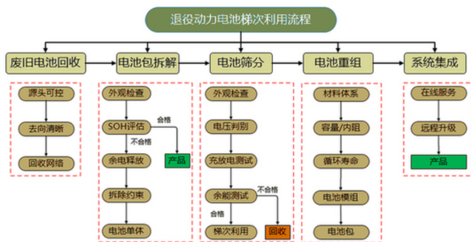
退役动力电池梯次利用流程
