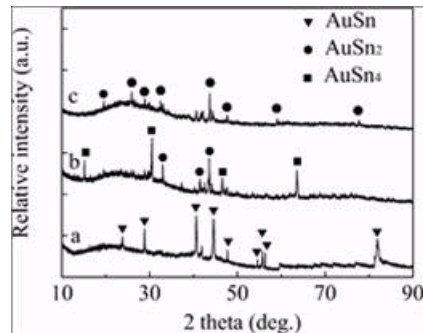
基于Au-Sn二元系中富Sn区域的圆片级局域加热键合及其中间层相组成
