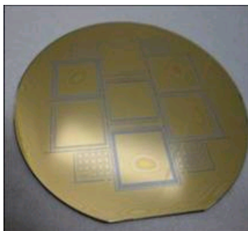
基于Au-Sn二元系中富Sn区域的圆片级局域加热键合及其中间层相组成
