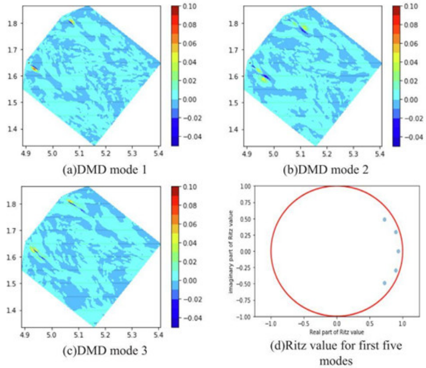
图2 前三阶动力学降解模式及其里茨图
