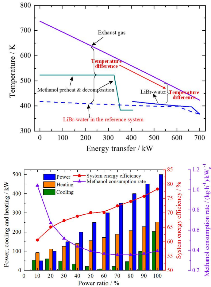
图2. 化学回热过程T-Q分析及分布式供能系统变工况性能 (白章, 刘启斌等, Applied Energy, 2018)
