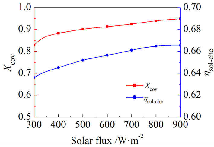
图1. 太阳能热化学燃料转化结构形式与其热力学性能 (刘泰秀, 刘启斌等, Applied Energy, 2018)
