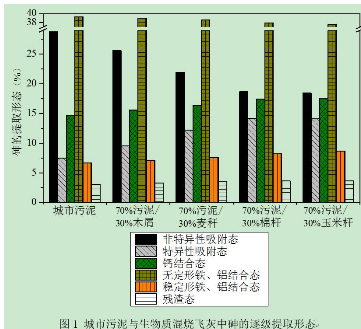
图1 城市污泥与生物质混烧飞灰中砷的逐级提取形态。
