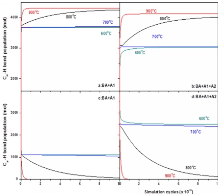
图2. B-M-P模型对煤共价键变化的预测
