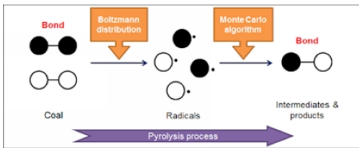
图1. 煤热解过程的“断裂-生成”机制
