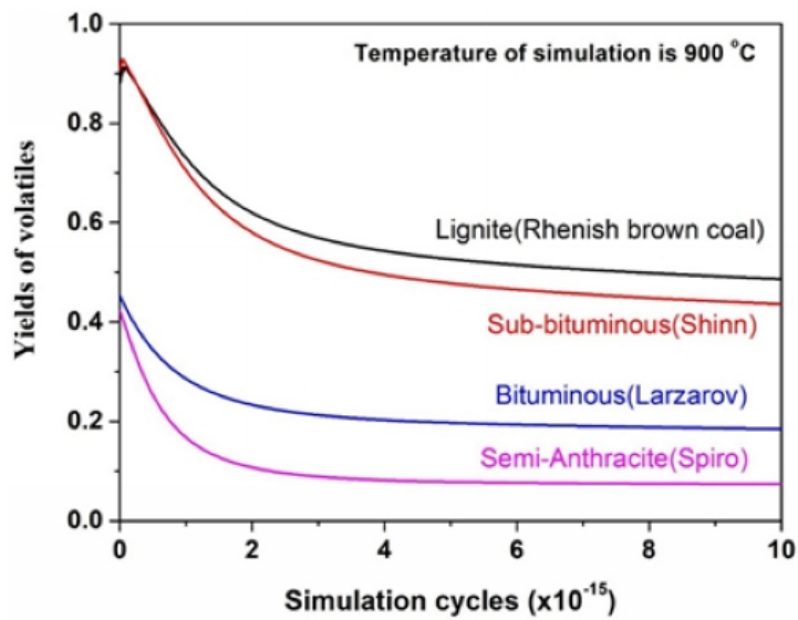
图3. B-M-P模型对不同煤挥发分产率的预测
