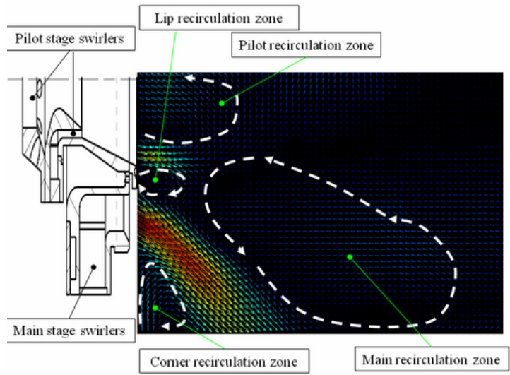
图2 分层部分预混新型燃烧室流场结构
