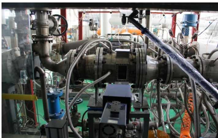
图1 高温高压雾化特性光学诊断实验平台
