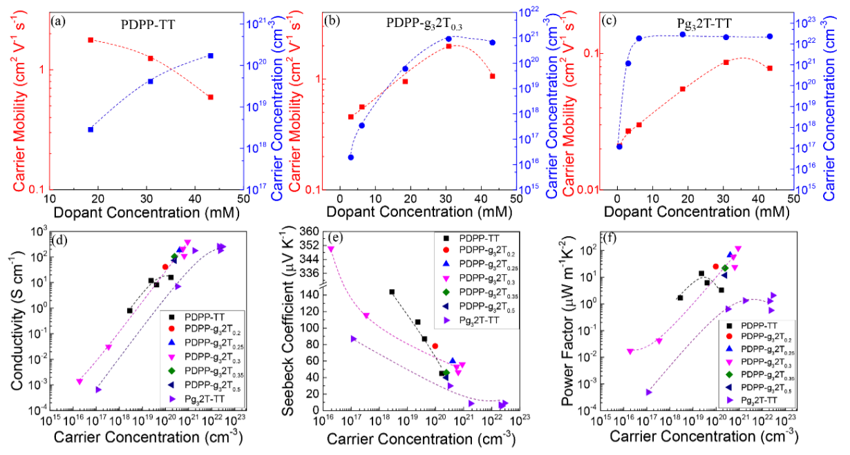
霍尔迁移率和载流子浓度随掺杂浓度的变化趋势以及聚合物热电性能
