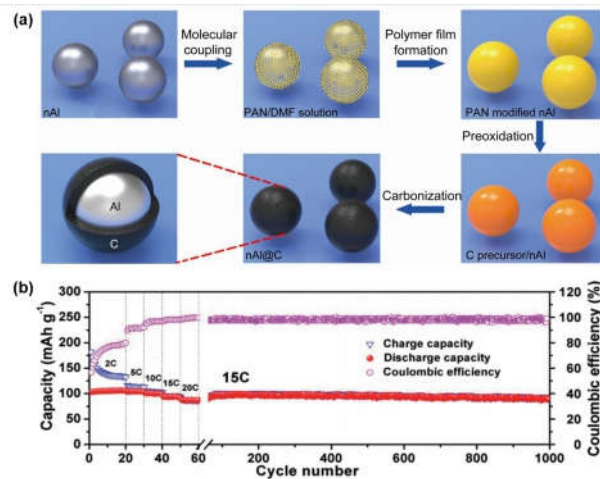
(a) 核壳结构铝@碳纳米复合材料的设计、制备示意图; (b) 所制备双离子电池在15C充放电速度下的长循环稳定性曲线。
