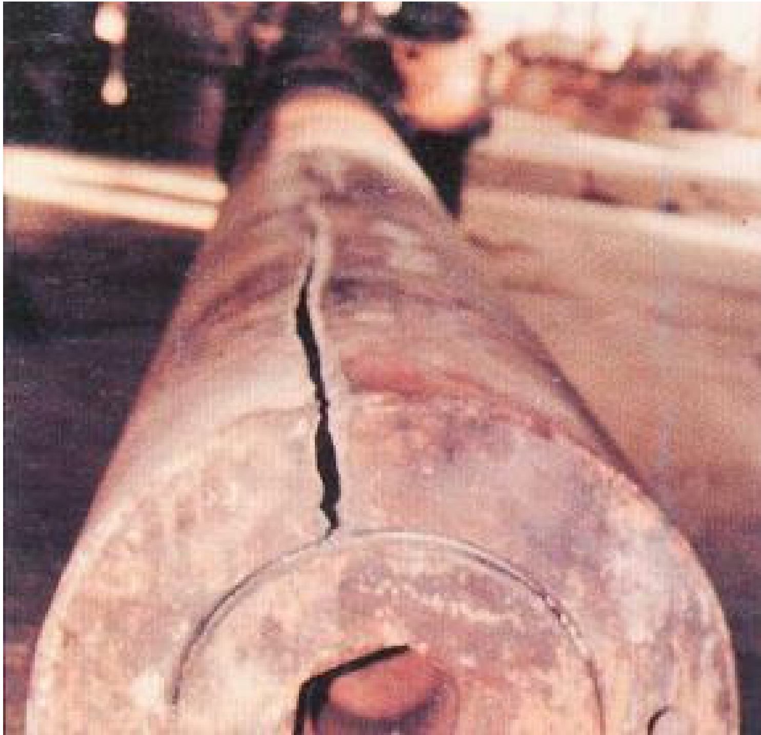
图2 厚壁容器 脆性断裂外观
