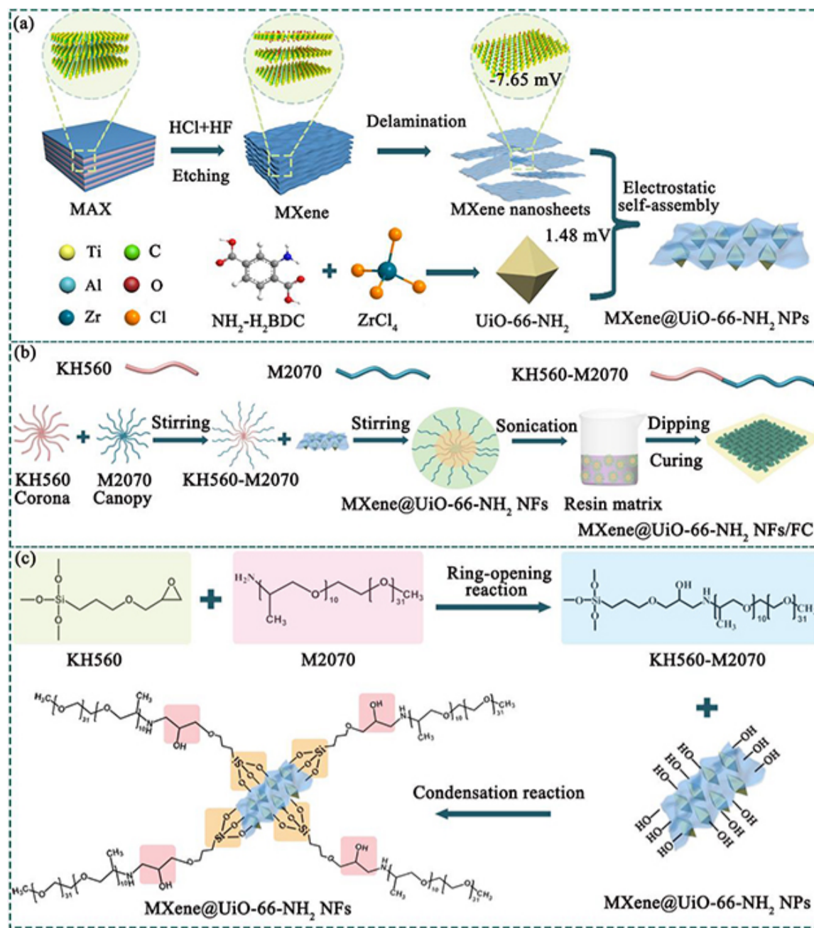
图1 MXene@UiO-66-NH 2 杂化纳米流体制备及反应机理示意图
