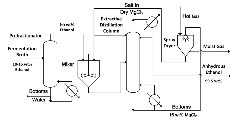
燃料乙醇脱水新工艺流程图
