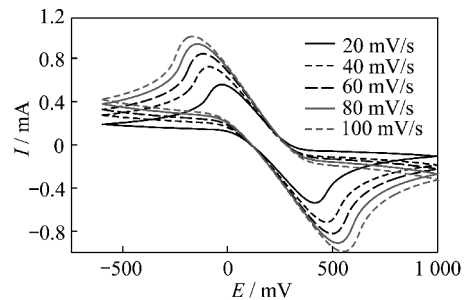
图3 不同扫描速率下离子液体的循环伏安曲线
