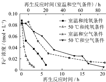
图 8 再生反应时间与 Fe 2+ 浓度的变化关系
