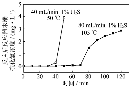
图5 不同反应温度下离子液体的脱硫穿透曲线
