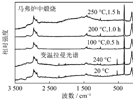
图1 离子液体随温度变化的拉曼光谱
