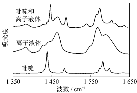
图2 吡啶与离子液体红外光谱
