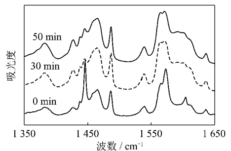
图6 反应前后氯化咪唑铁基离子液体与吡啶混合物的红外光谱
