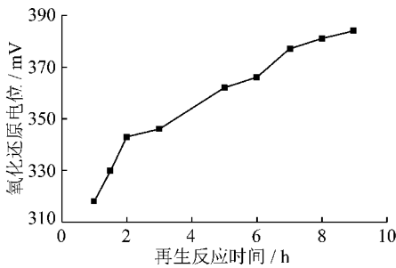
图 7 再生反应时间与氧化电位关系
