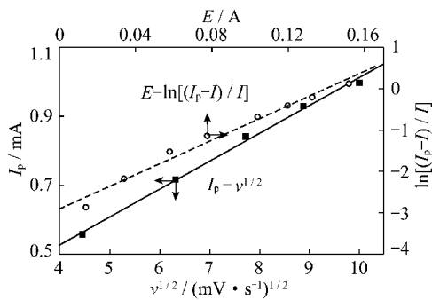
图4 离子液体峰电流、电压及扫描速率关系
