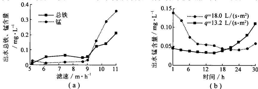
图 2 滤速和反冲洗强度对出水水质的影响
