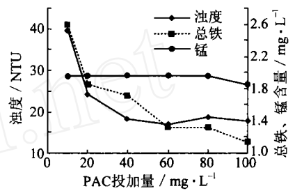
图 1 投药量对混凝沉淀效果的影响
