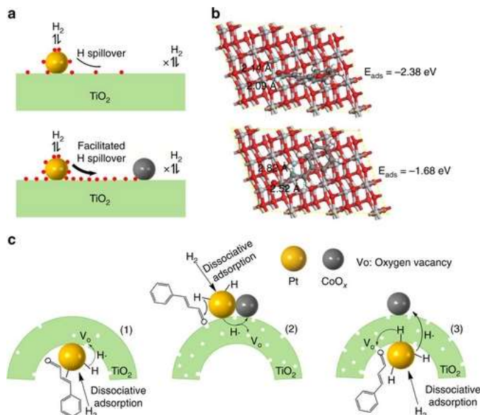
图3. (a) CoO x 对TiO 2 负载Pt催化剂的氢溢流机制的影响; (b) C=O及C=C在TiO 2 的空氧位 (O v ) 上的吸附强度DFT模拟计算结果; (c) 肉桂醛加氢反应选择性增强机制。
