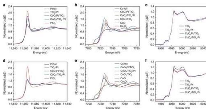
图2. 催化剂非原位 (a) 和原位 (d) Pt L 3 边XANES图; 催化剂非原位 (b) 和原位 (e) Co K边XANES图; 催化剂非原位 (c) 和原位 (f) Ti K边XANES图。
