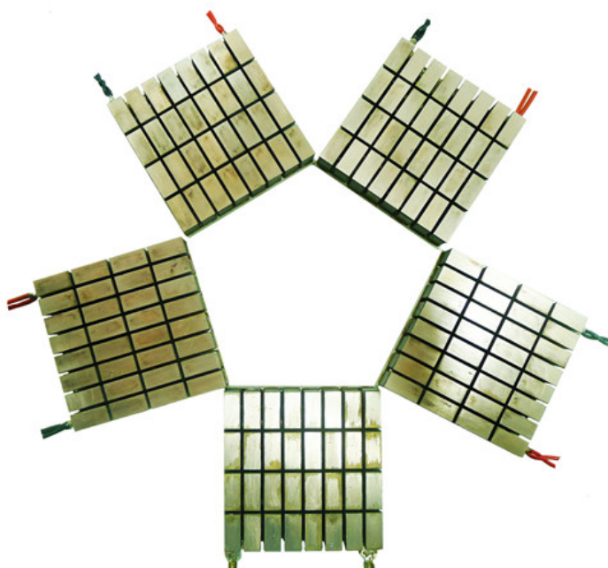
图2. 方钴矿基笼状化合物热电发电器件。
