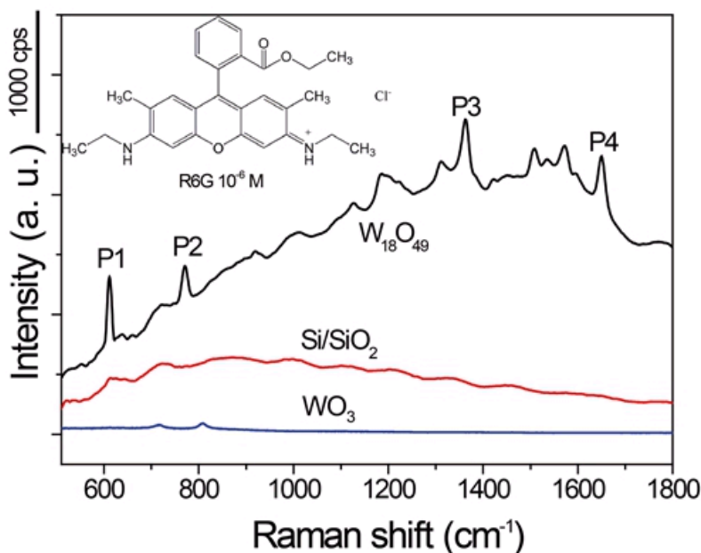
富氧缺陷的 W_{18}O_{49} 纳米粒子作为SERS基底性能优秀
