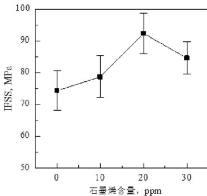
图3 石墨烯含量对碳纤维复合材料IFSS性能的影响
