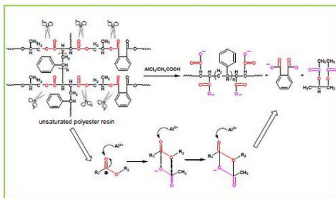
图2. 选择性断裂酯键降解回收玻纤/不饱和聚酯复合材料
