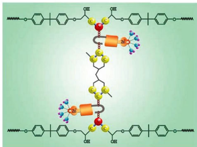
图1. 选择性断裂碳氮键降解回收碳纤/环氧复合材料
