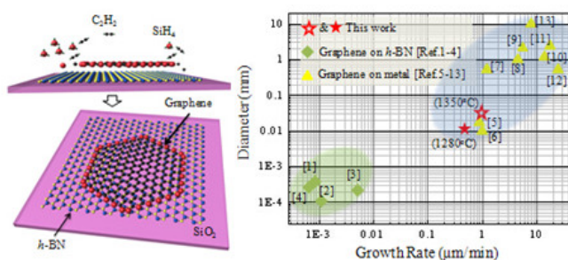
气相催化法生长石墨烯单晶的示意图（左）和所得单晶尺寸和生长速率与之前文献报道数据比较（右）
