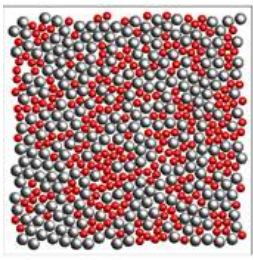
硬球胶体玻璃瞬时位形图（左）和相图（右）。
