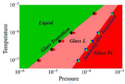
硬球胶体玻璃瞬时位形图（左）和相图（右）。
