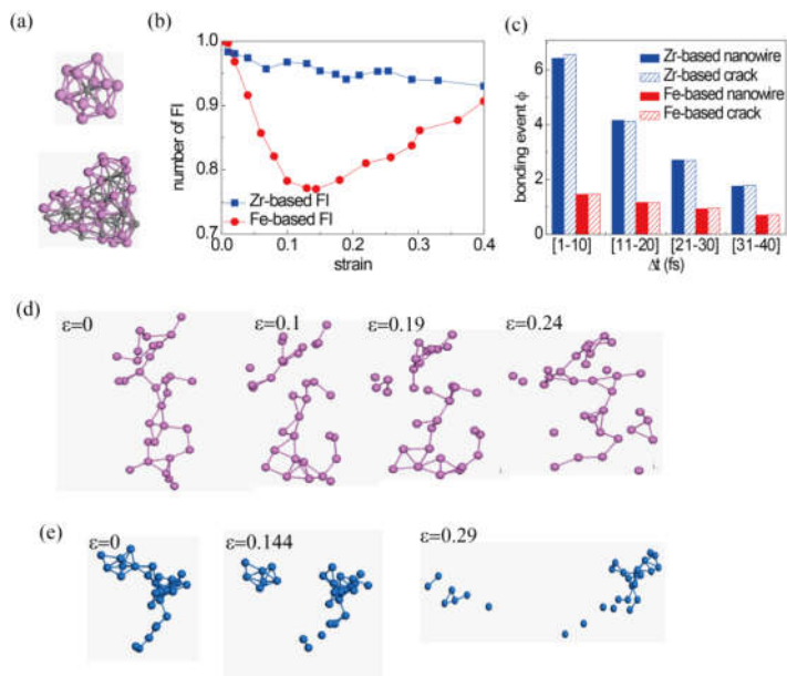
图2: (a) 原子团簇组成的正二十面体以及多个团簇组成的示意图。(b) 加载过程中Zr基和Fe基团簇数目的变化。(c) 团簇自愈能力的比较。(d) 加载过程中Zr基团簇自愈示意图。(e) 加载过程中Fe基团簇断裂示意图。
