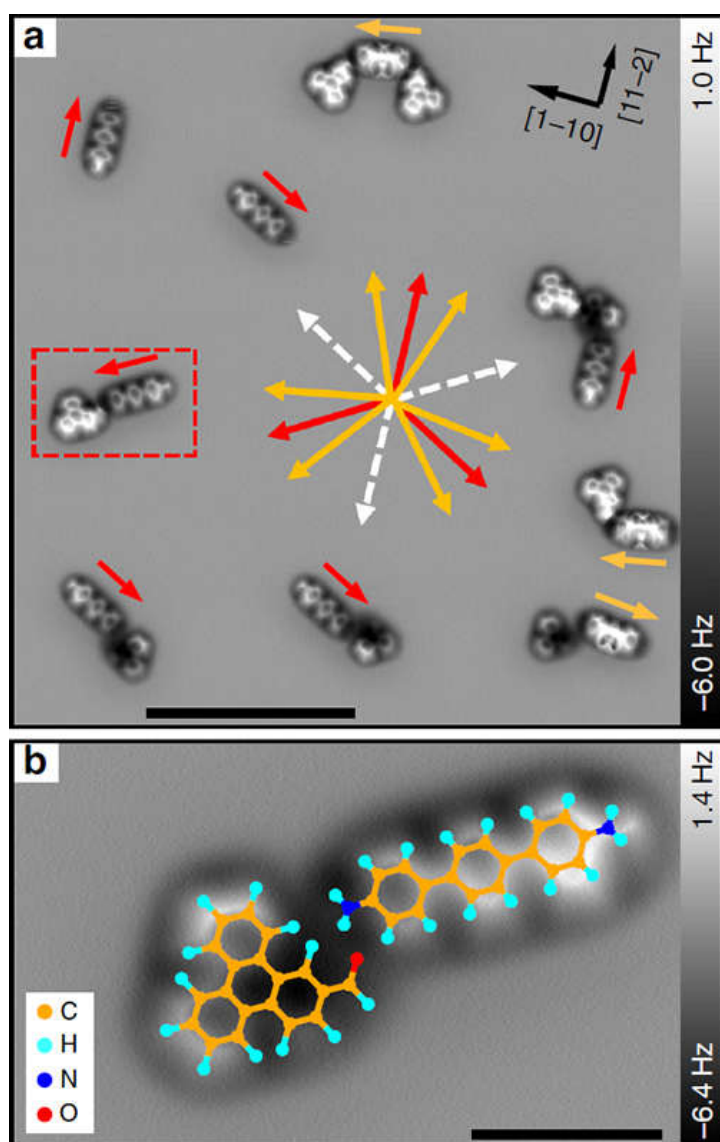
图5. DATP和TPCA分子的自组装。
