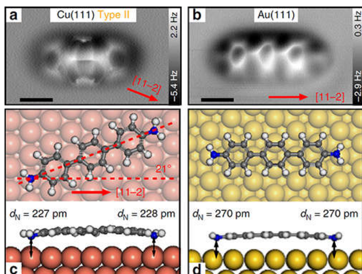
图4. DATP分子在Cu(111)和Au(111)表面上的第二种对称的吸附构型。
