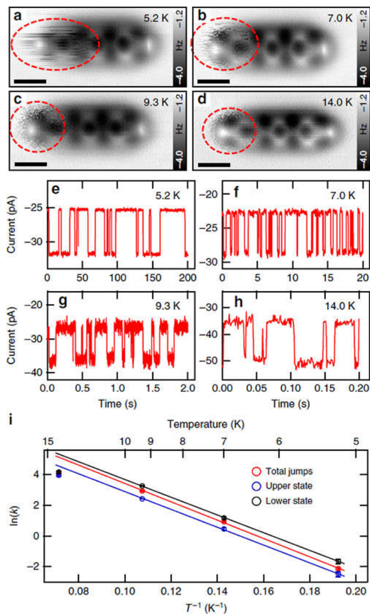
图2. 观测到的跳跃机制的动力学分析和能量势垒。
