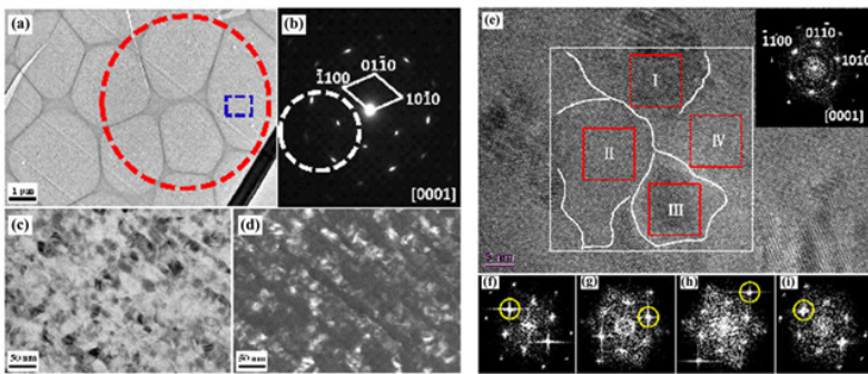
图2. 马赛克晶体热电材料的微观结构
