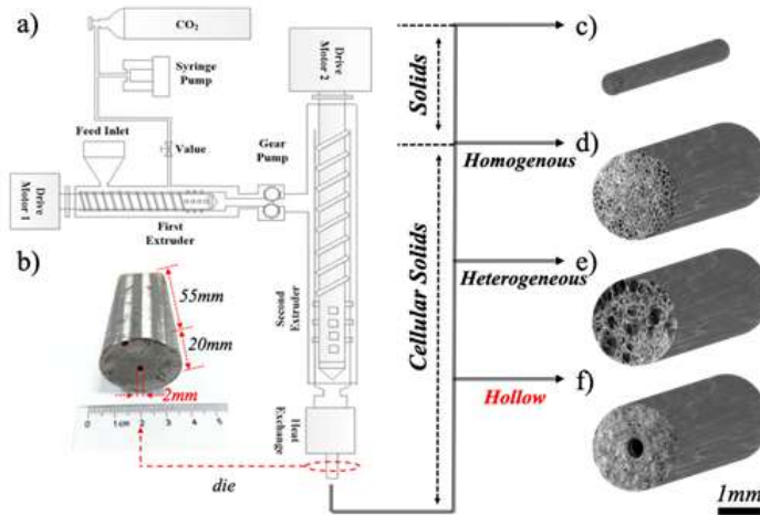
图1 一样的挤出机，不一样的结构
