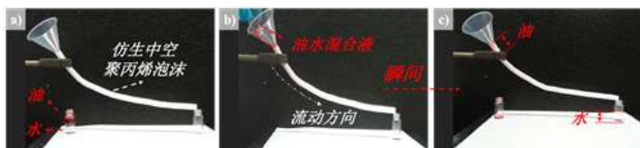
图3 进的是油水混合液，出的是水
