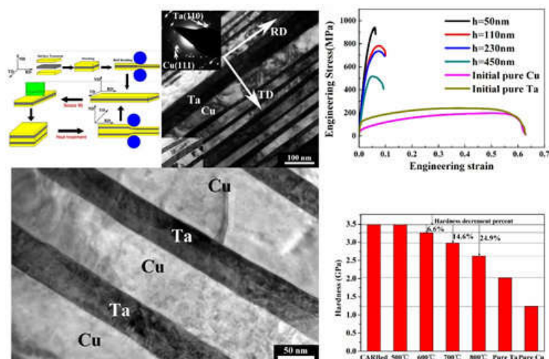
图：CARB工艺制备的层厚为50nm Cu/Ta纳米多层膜块体微观结构、力学性能及热稳定性
